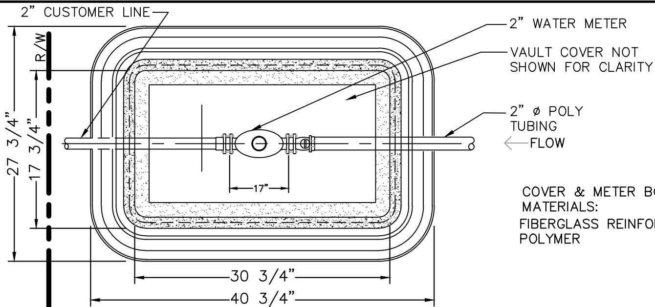
PLAN N.T.S.
