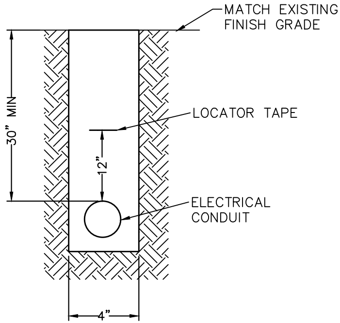
ELECTRICAL CONDUIT IN EARTH N.T.S (TYP.)
