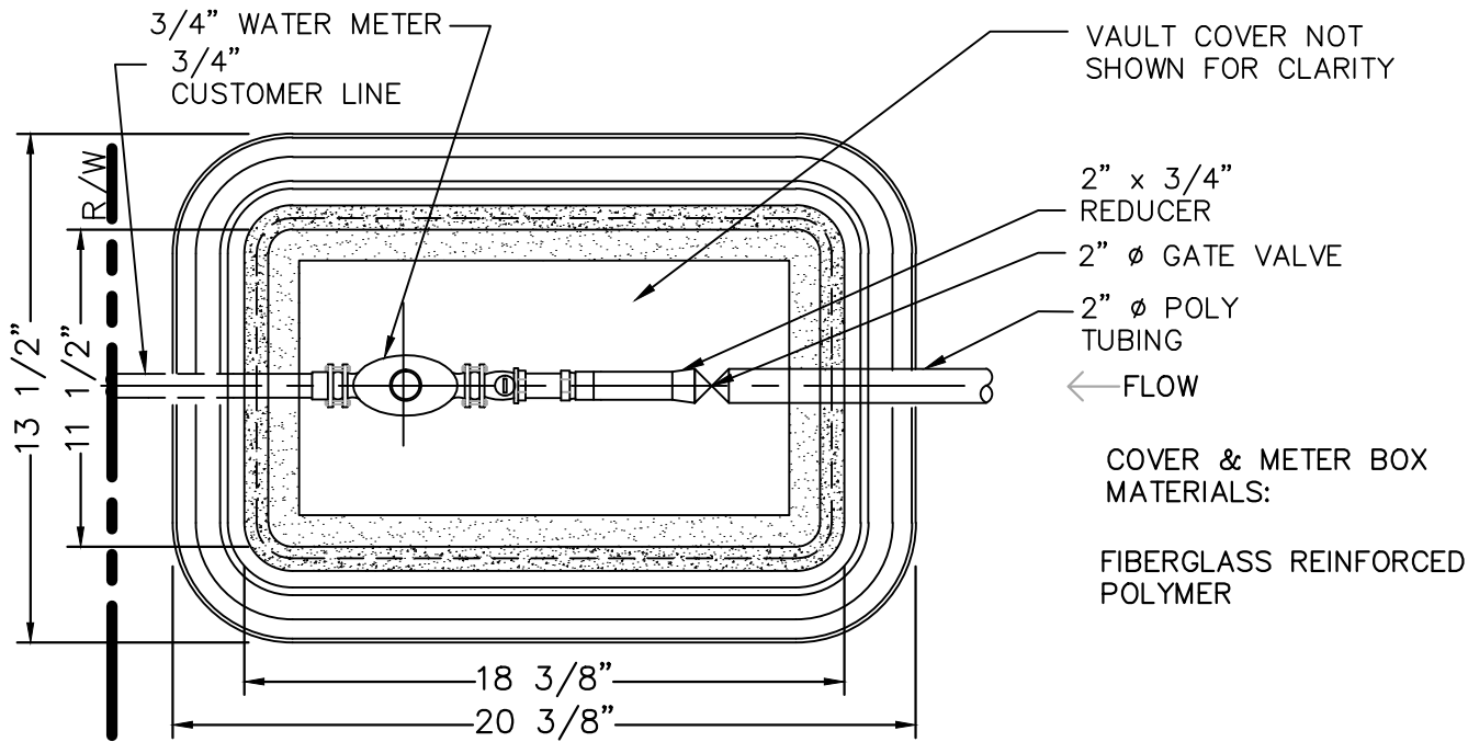
PLAN N.T.S.
