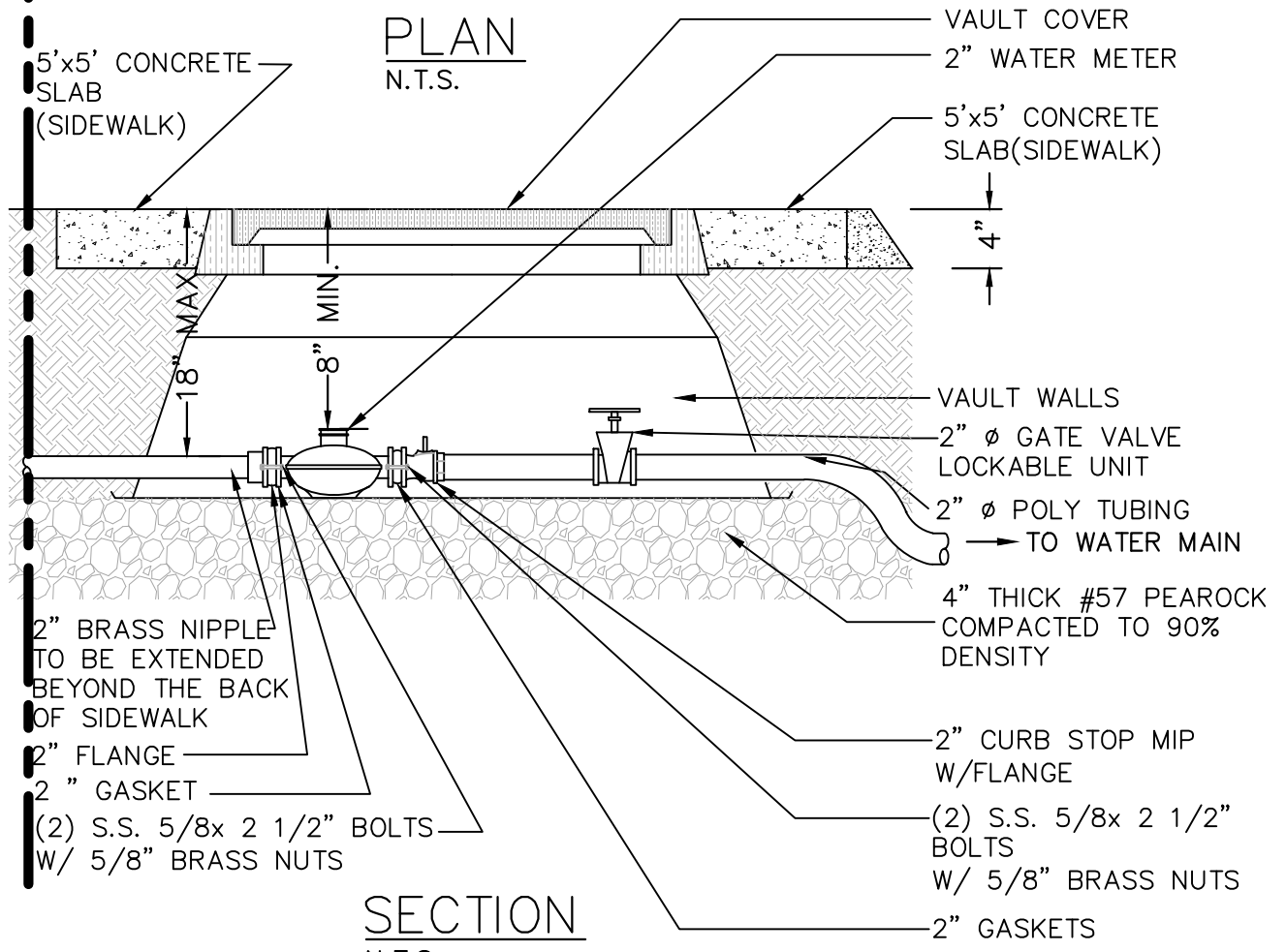
2" WATER METER DETAIL N.T.S.
