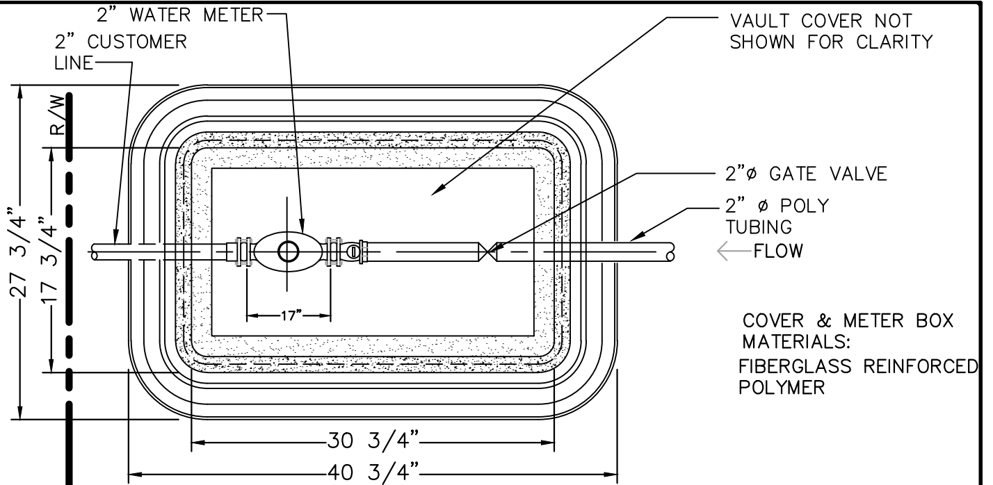
PLAN N.T.S.
